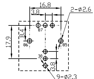
常开型 1 Form A
