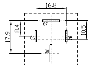
常开型 1 Form A
