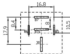
转换型 1 Form C
